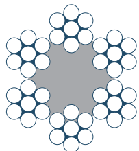
6 x 7 + AF 1 + 6
