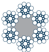
6 x 19 + AF Seale 1-9-9
