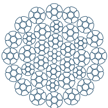
35x7 1+6
