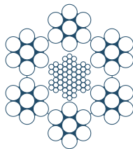
6 x 7 + AACI 1 + 6
