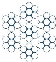
6 x 7 + AA 1 + 6
