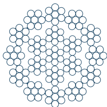
19 x 7 1+6
