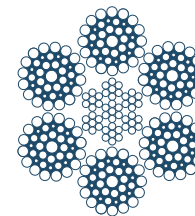
6 x41WS-AACI WS 1-8-8*8-16
